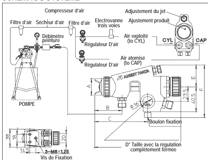
SCHÉMA DU SYSTÈME
