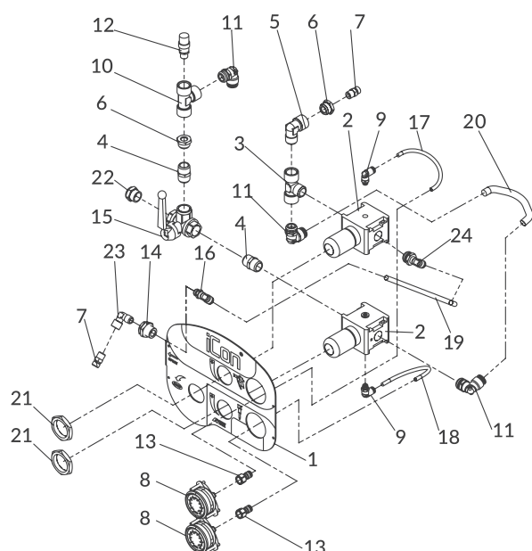
Régulateur d'air
