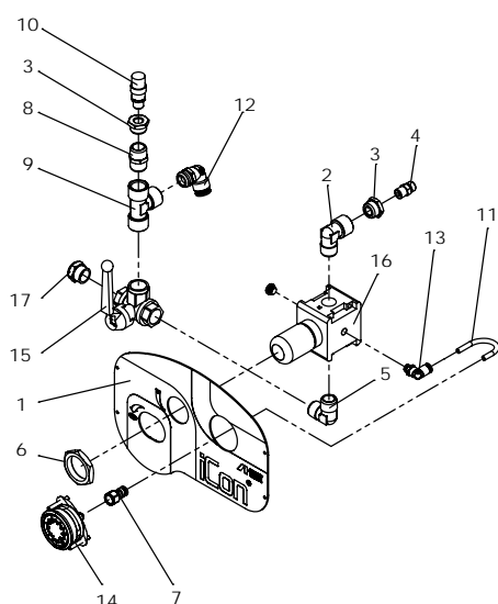
Distributeur d'air
