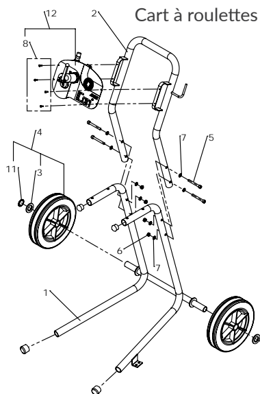
Cart à roulettes
