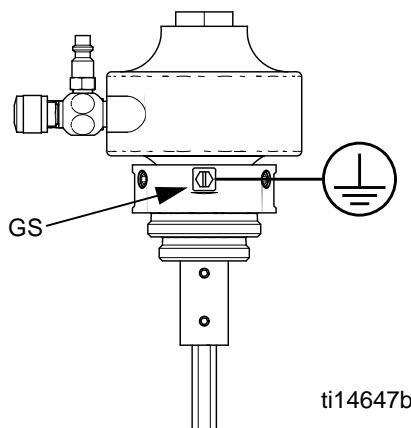
FIG. 1: Vis de mise à la terre
