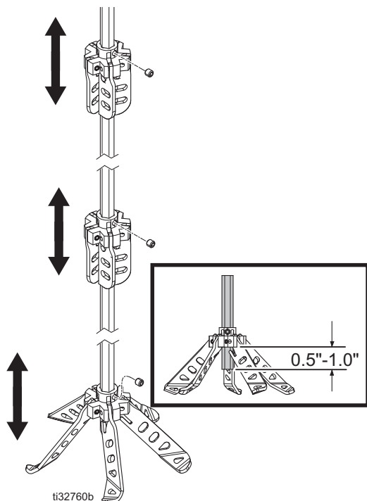
FIG. 3: Réglage de la place des ensembles moyeu/lame
